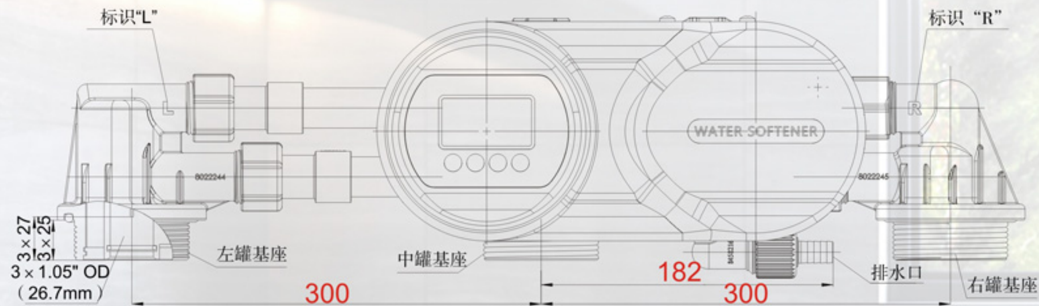
18601B(F120B) 693×258×152mm
