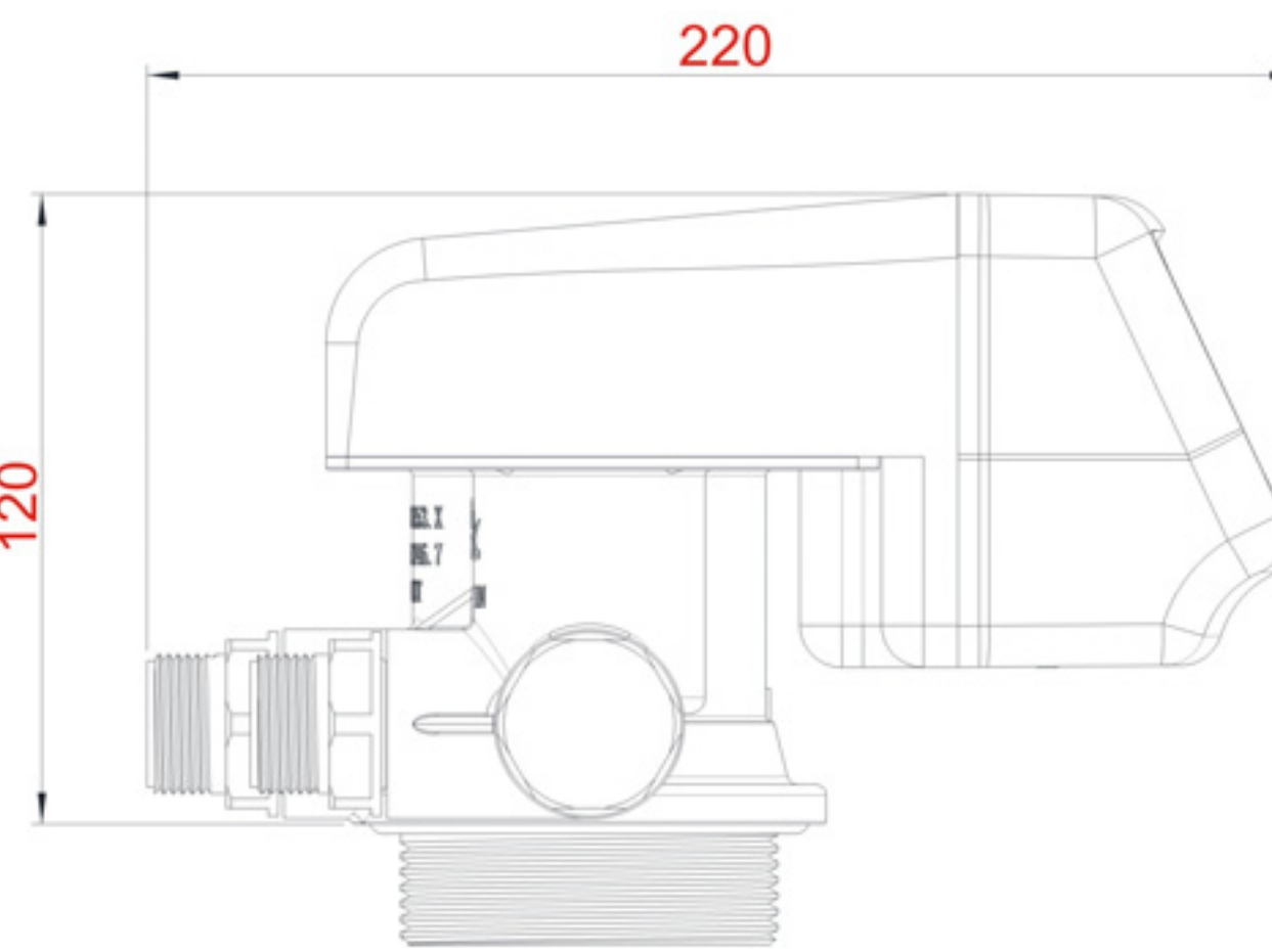
52502(F71D1) 220 × 199 × 120mm
