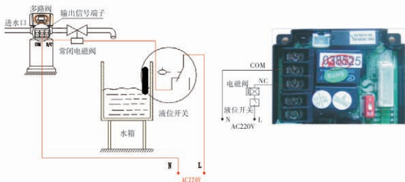
图3-1 控制出口电磁阀的接线图
