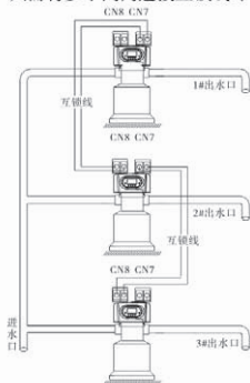
图3-12 同时供水，分别再生
