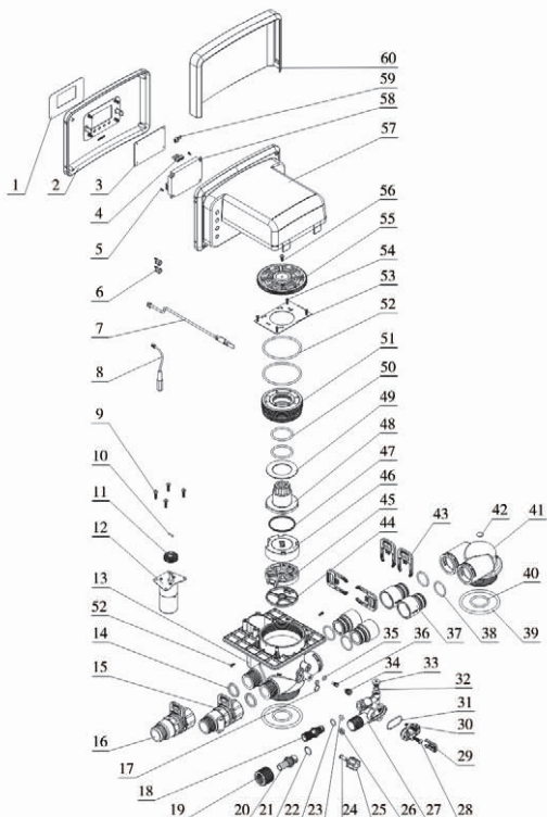
F142A3/F142B3的结构图
