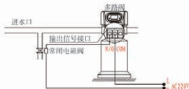
图3-3 泄压端口的接线图
