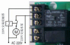
图3-8进口接增压泵的接线图
