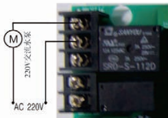
图3-7 进口接增压泵的接线图
