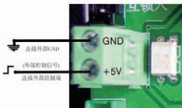
图 3-11 远程控制端口的接线图
