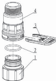
5457002活接头
