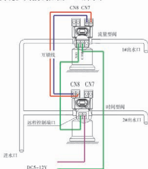
图3-13 同时供水，顺序再生
