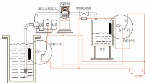
图3-5 通过水箱液位控制进水泵的接线图
