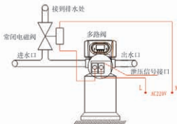
图 3-10 泄压端口的接线图
