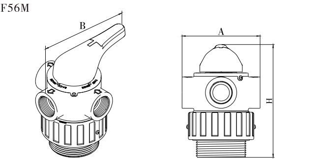
外形尺寸
