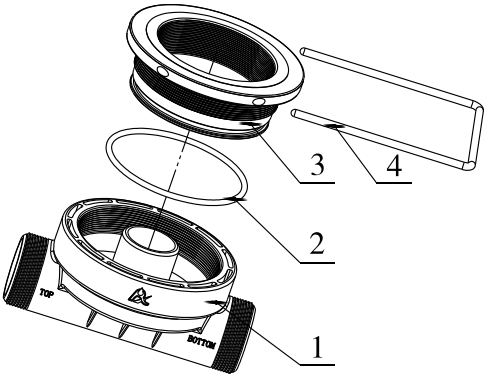
5458002侧装连接件名称及编码:
