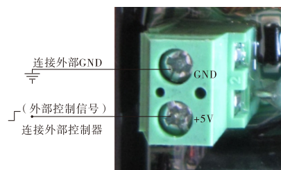
图3-11 远程控制端口的接线图
