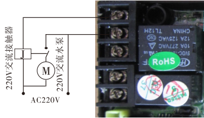
图3-8 进口接增压泵的接线图
