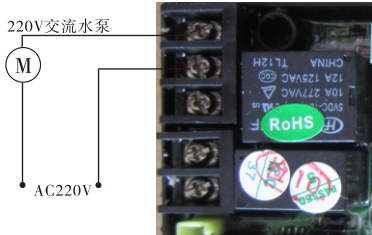
图3-7 进口接增压泵的接线图
