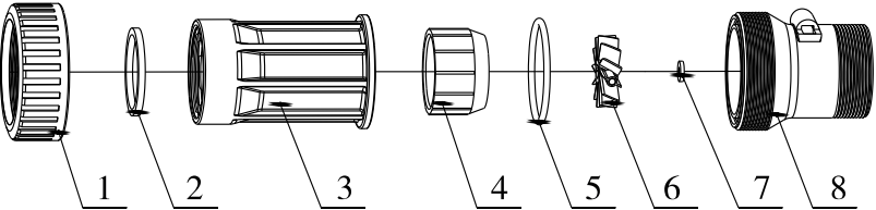
5447003流量计结构图:
