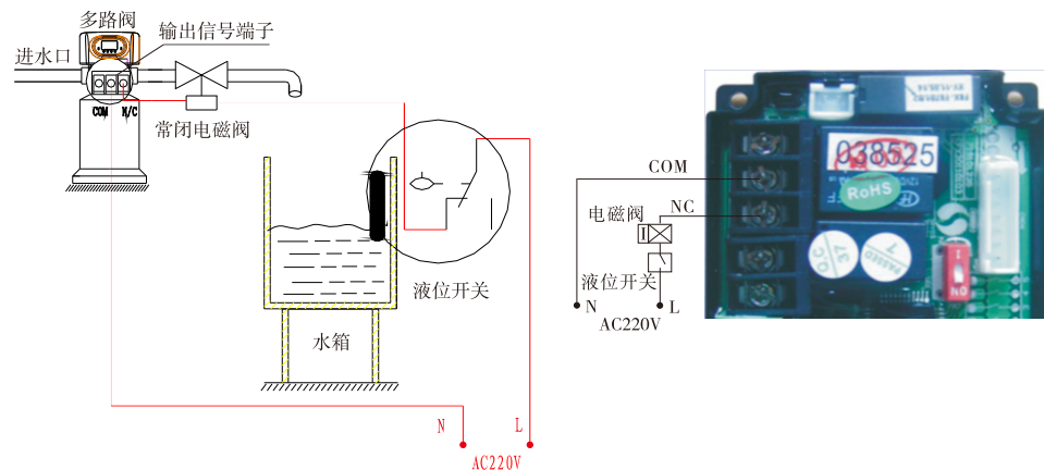
图3-1 控制出口电磁阀的接线图
