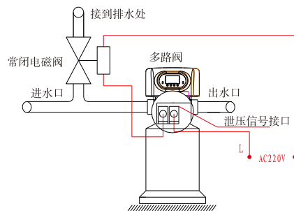
图3-10 泄压端口的接线图
