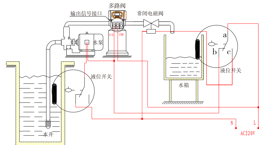
图3-5 通过水箱液位控制进水泵的接线图
