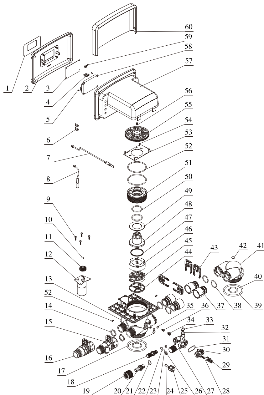
F142A3/F142B3的结构图
