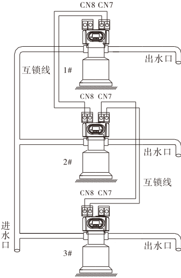
图3-10 同时供水，分别再生
