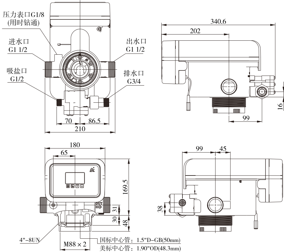
63508/63608结构图
