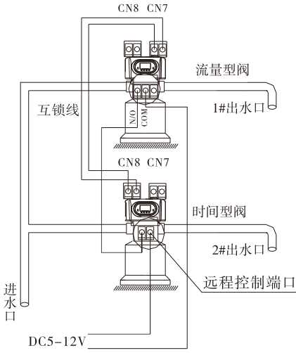
图3-11 同时供水，顺序再生
