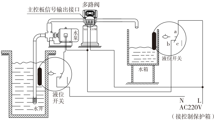
图3-4 通过水箱液位控制进水泵的接线图
