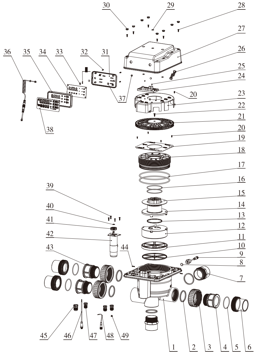
F152C的爆炸图：
