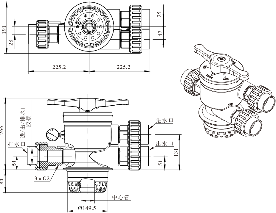
F139AS结构图
