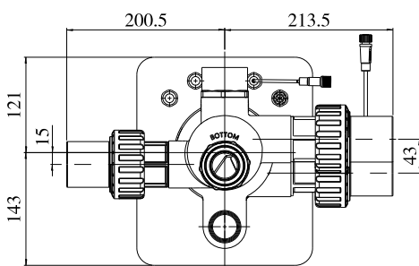
F139C结构图
