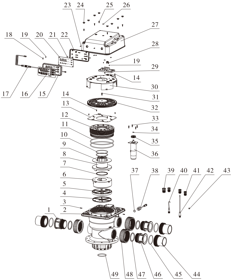
F152B-1结构图：
