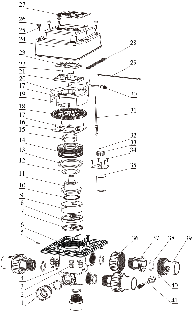
F138C结构图:
