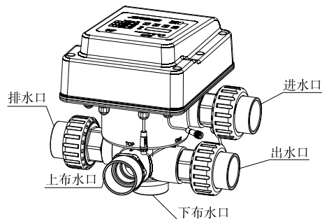
F139C结构图
