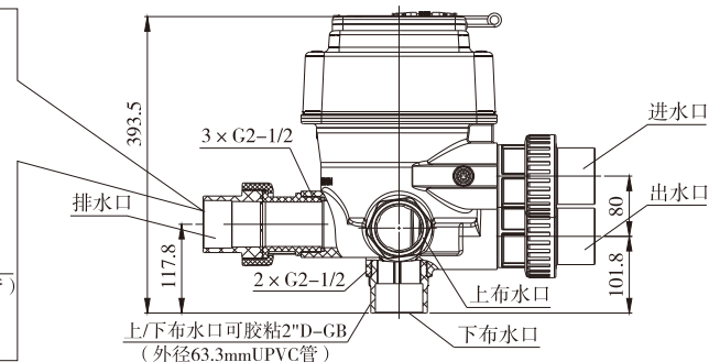
F152C结构图
