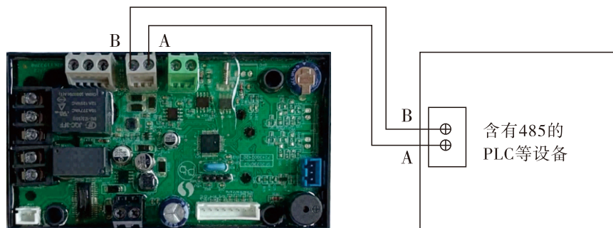
图3-4 单台阀与PLC等设备485接线图
