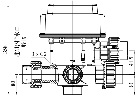
F139C结构图
