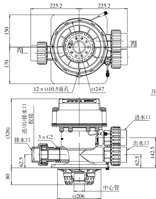
F139B-3结构图
