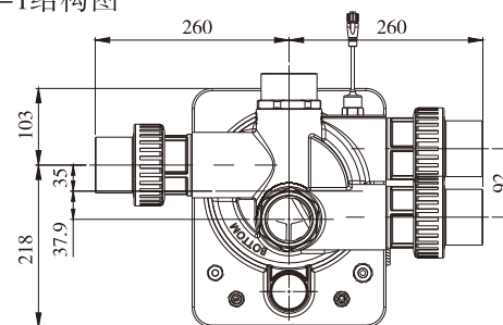
F152B-1结构图
