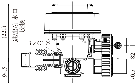
F138C结构图
