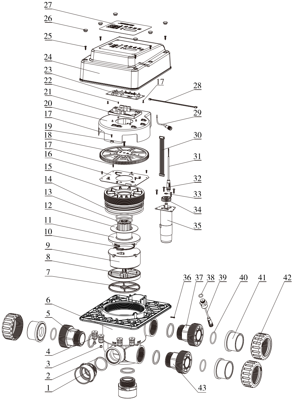
F139C结构图:
