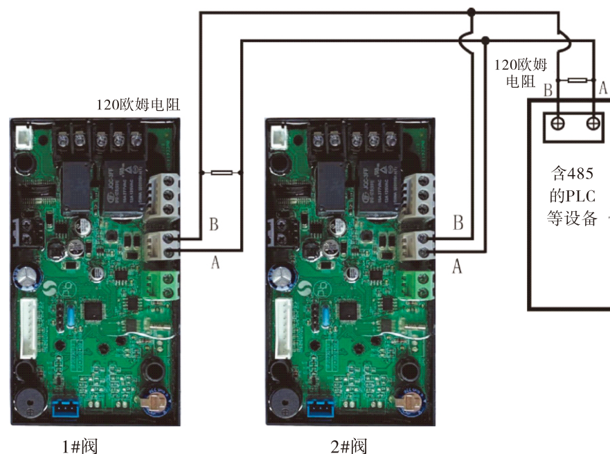
图3-5 多台阀与PLC等设备485接线图
