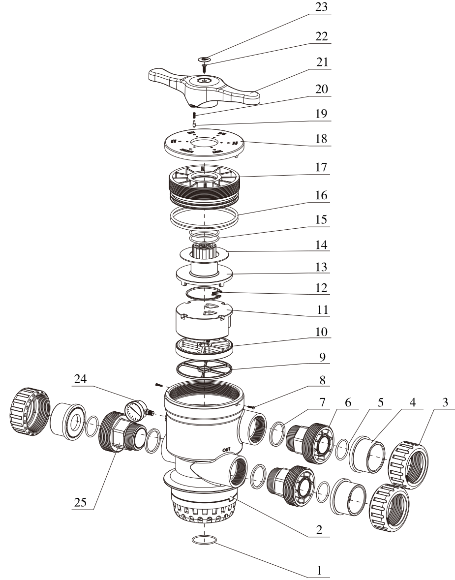
F139S结构图:
