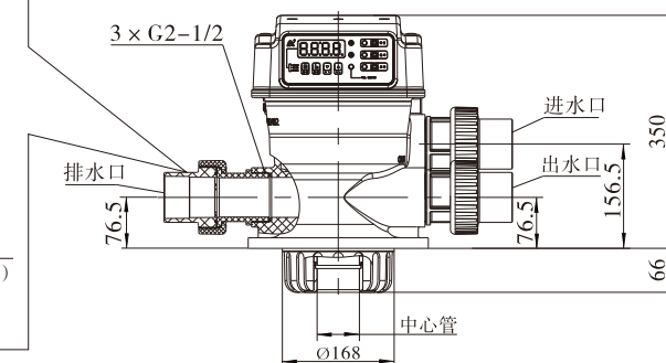
F152B-1结构图
