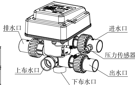
F138C结构图
