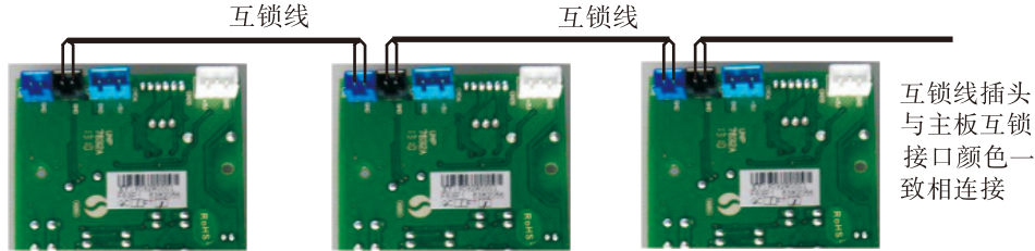
图3-9 互锁的接线图
