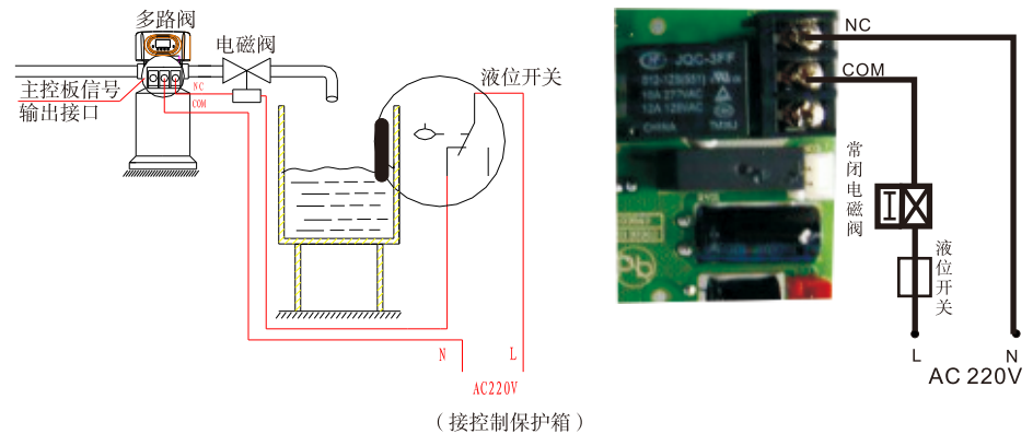
图 3-1 控制出口电磁阀的接线图
