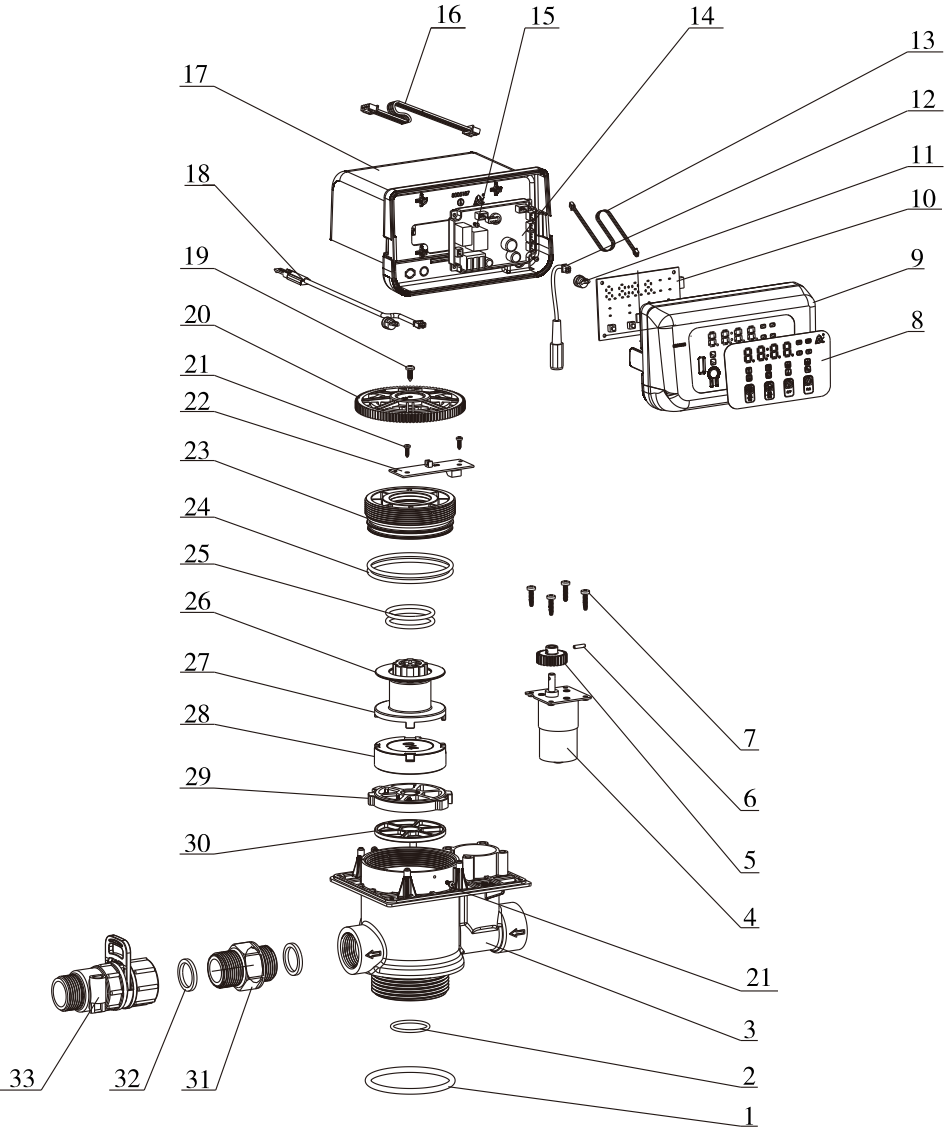
F67S3爆炸图
