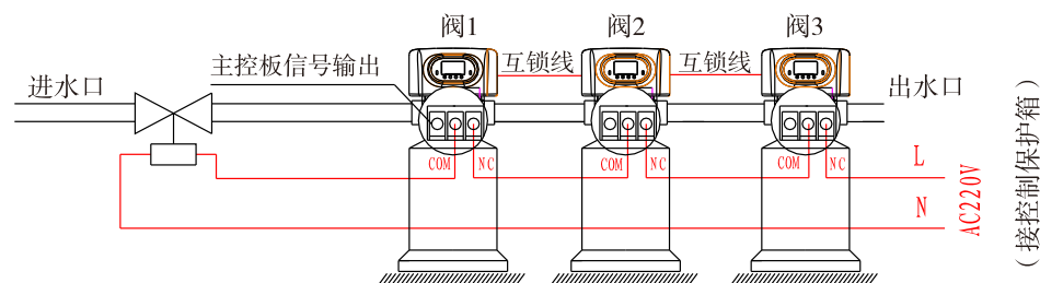
图3-4 多级串联时控制进口电磁阀的接线图
