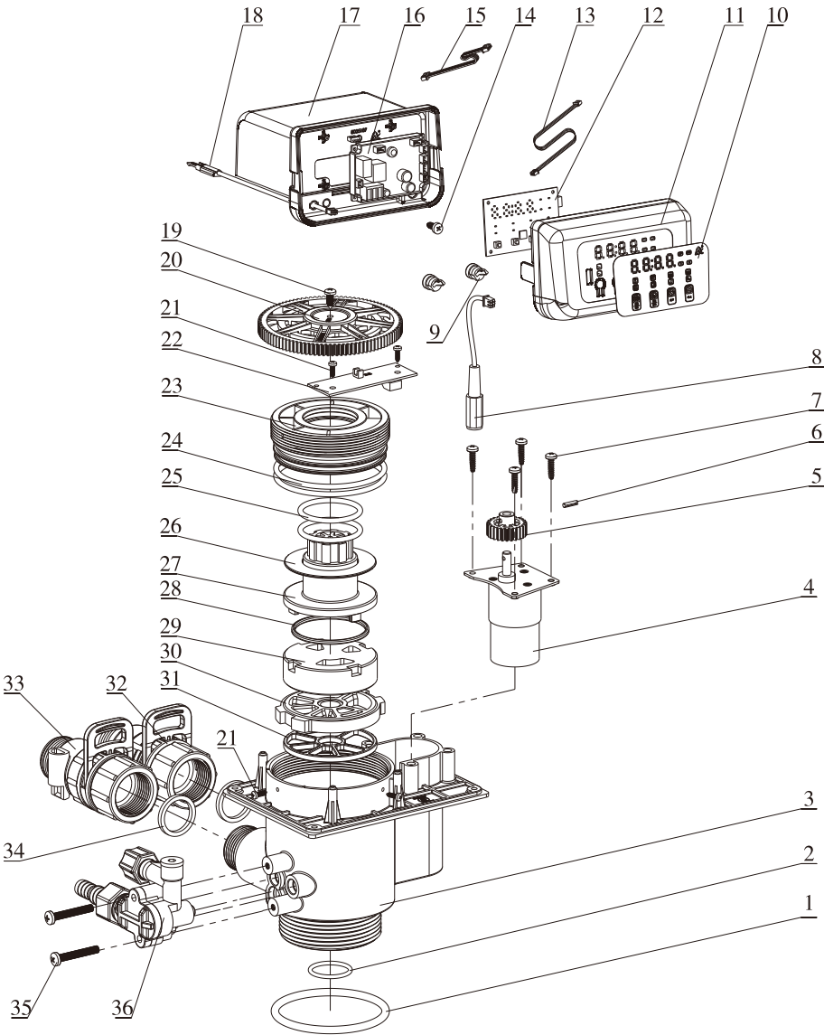
F63S3爆炸图
