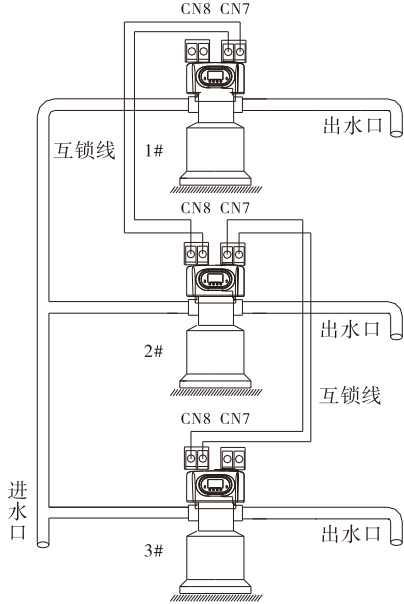
图3-10 同时供水，分别再生
