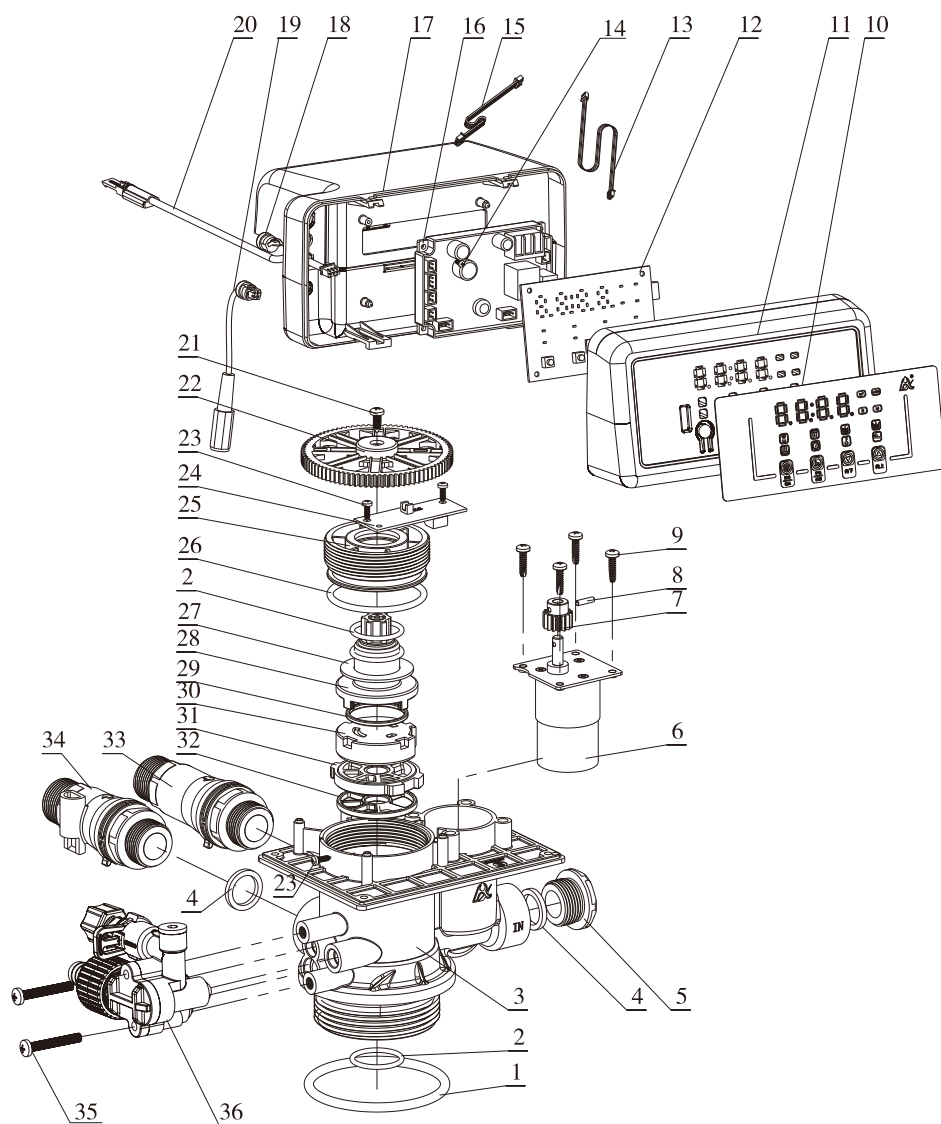
F65S3爆炸图
