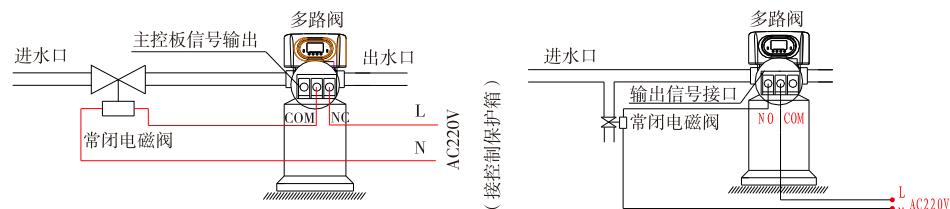
图3-2 控制进口电磁阀的接线图
